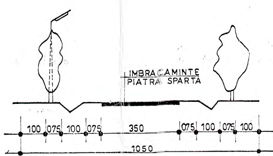
PROFIL TRANSVERSAL STRAZI ULITE 4 - 4
